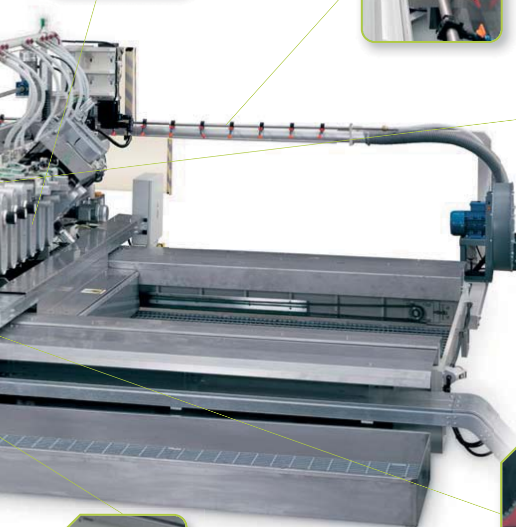
Barra intermedia automatica per vetri di grandi dimensioni. Automatic intermediate bar for big-sized glasses. Automatische Mittenunterstützung bei großen Glasabmessungen. Barra intermedia automática para grandes hojas de vidrio. Barre intermédiaire automatique pour verres de grandes dimensions.
